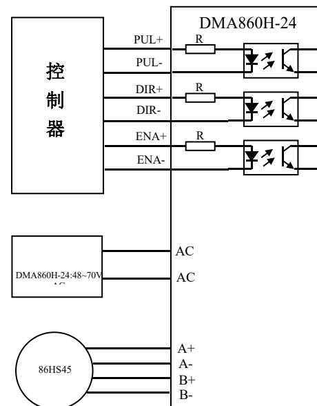
图 6. DMA860H-24 配 86HS45 典型接法
