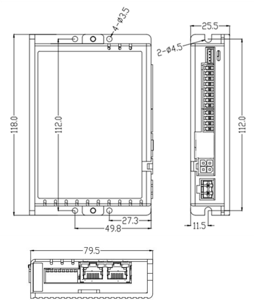
图 2-1 DM2C-RS522/556/870 系列驱动器机械尺寸
